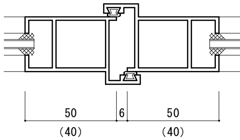
両開き召合せ
