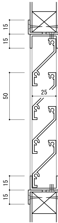
角ガラリ
