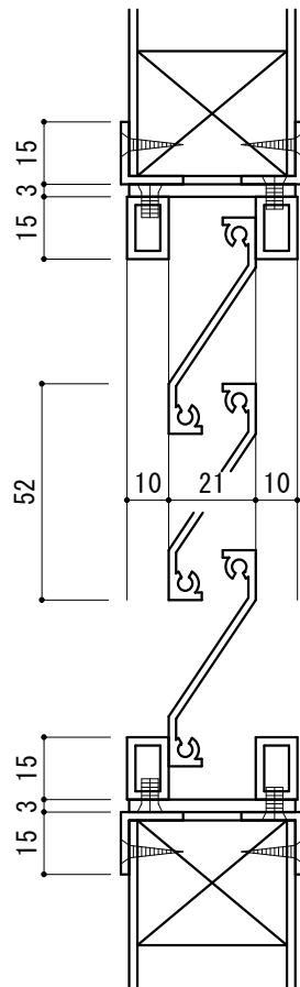
三角ガラリ
