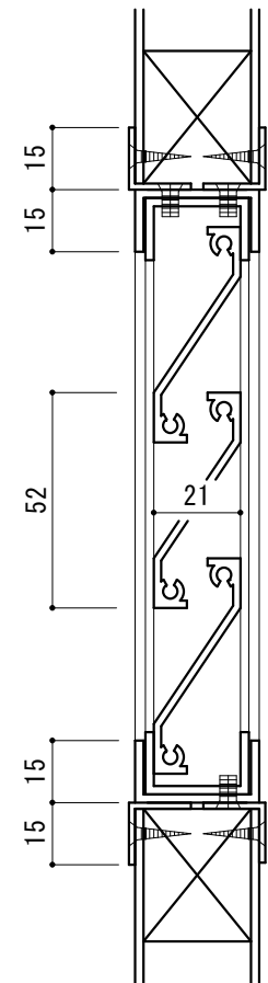
丸ガラリ
